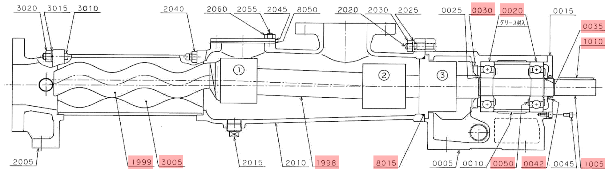
一軸ねじ式ポンプNE型組立断面図
