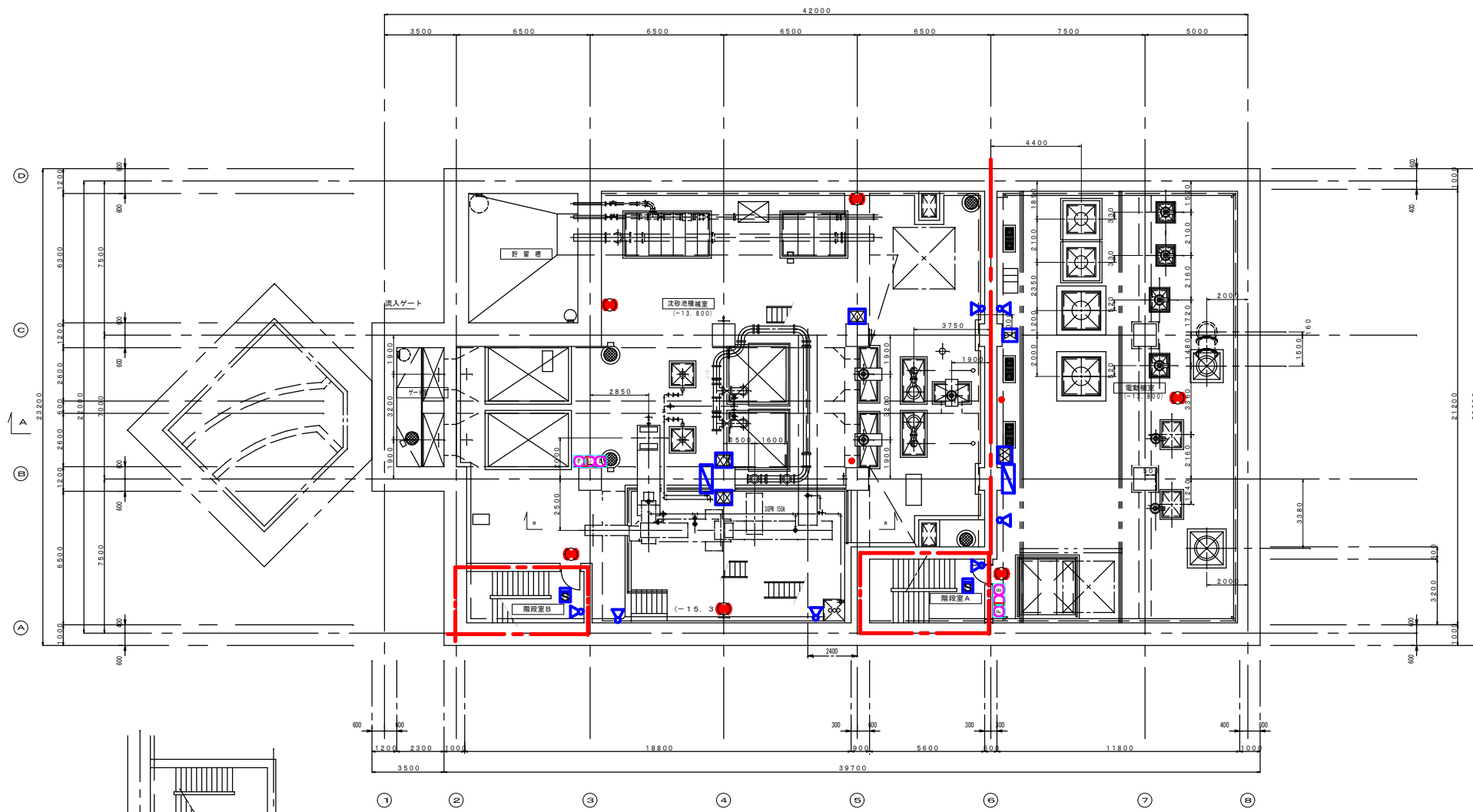
地下2階下部平面図 1/200
