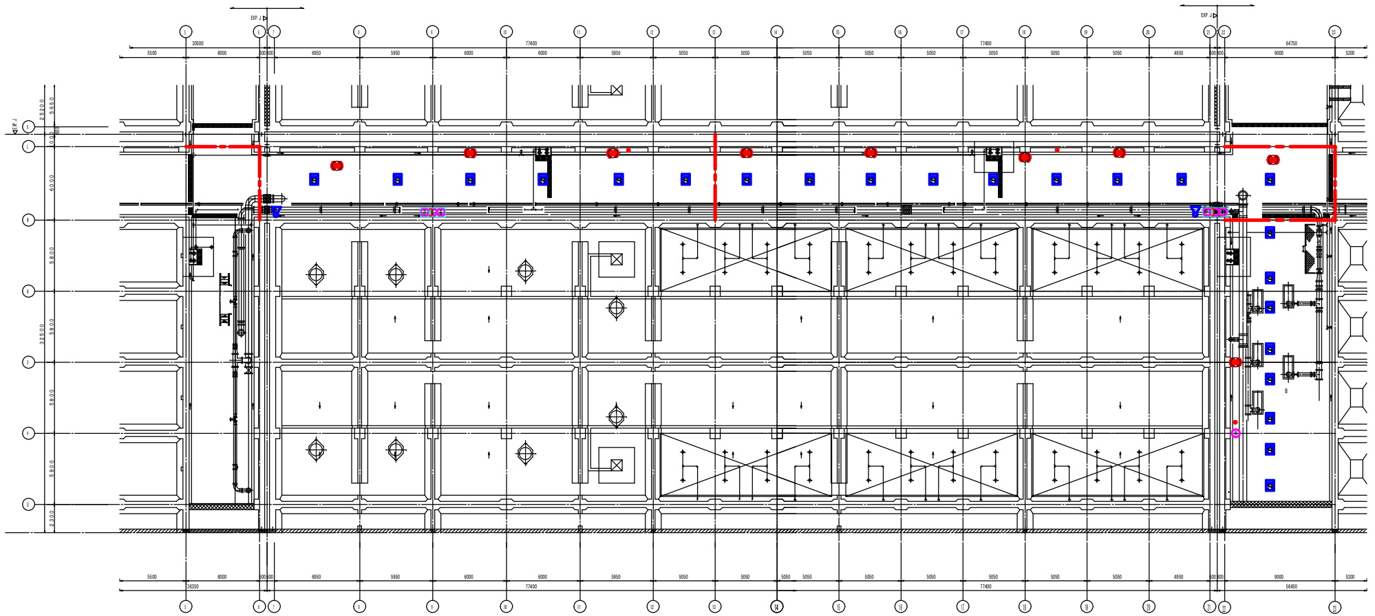
2系水処理反応平面図 S=1/300
