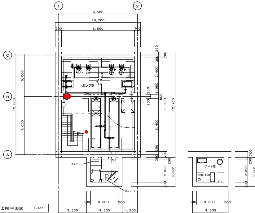
B 2階平面図 1/100
