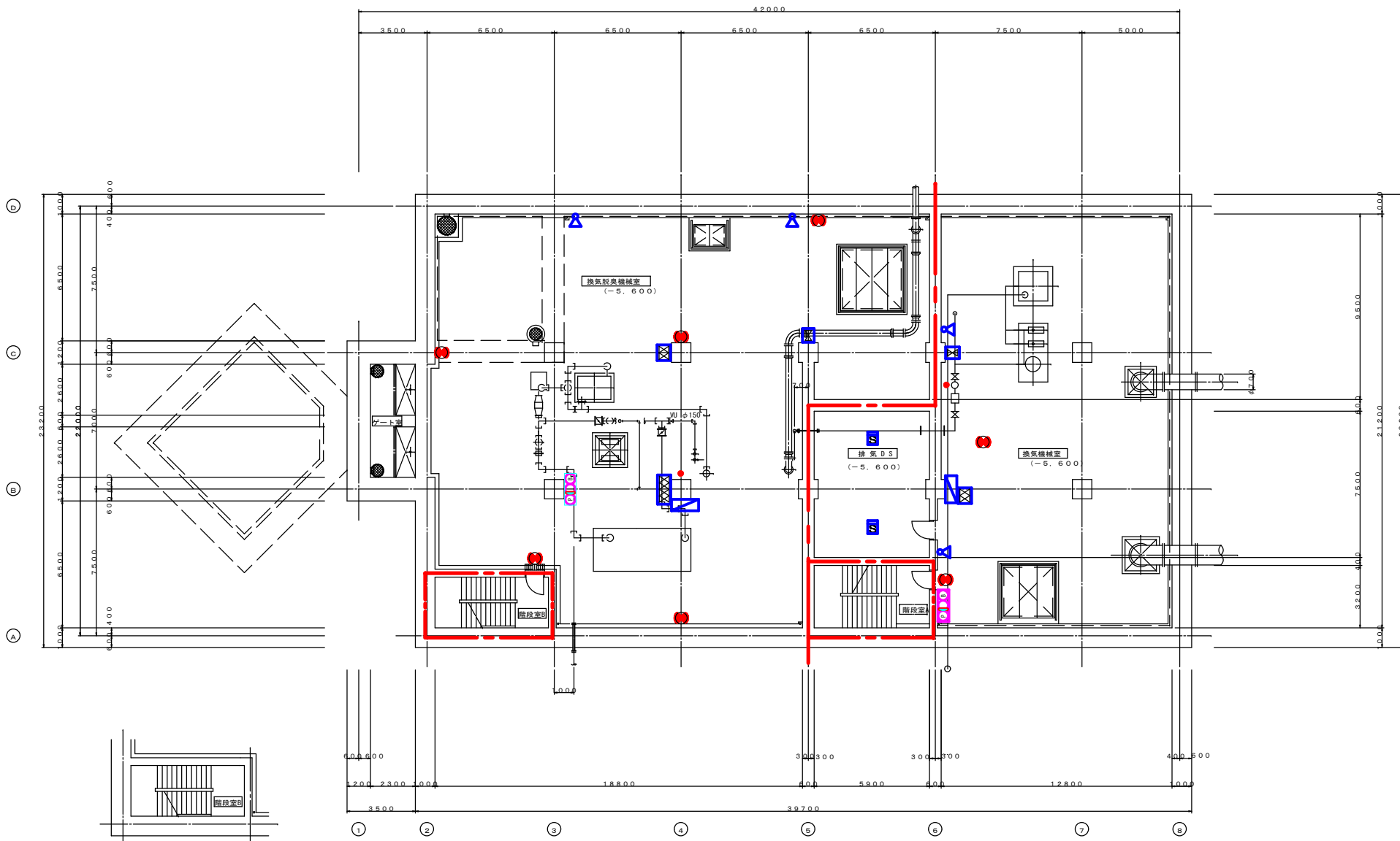
地下1階平面図 S=1/200
