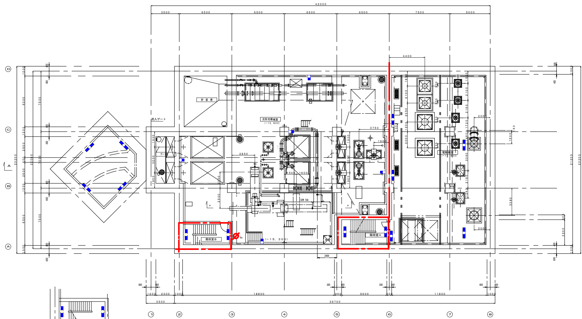
地下2階下部平面図 1/200
