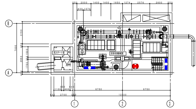
地下1F平面図 S=1/200
