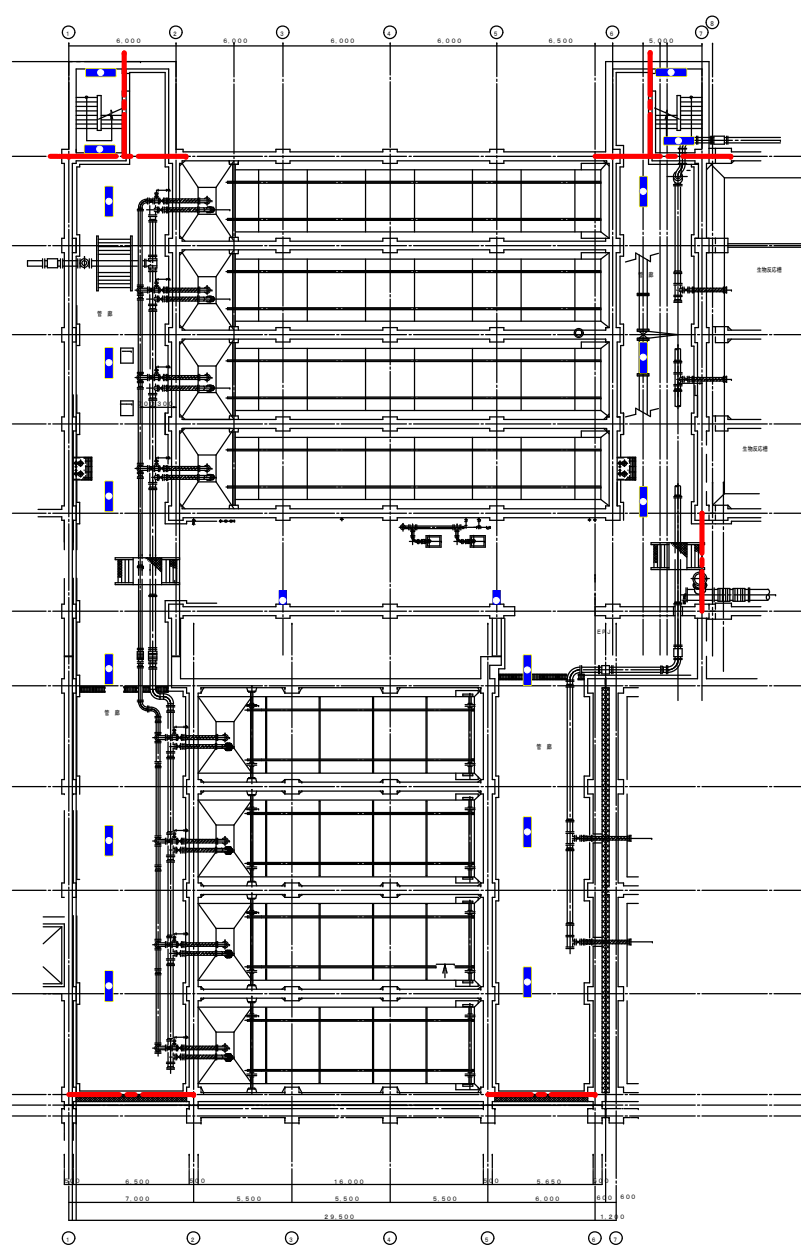
初設下層平面図 S=1/300
