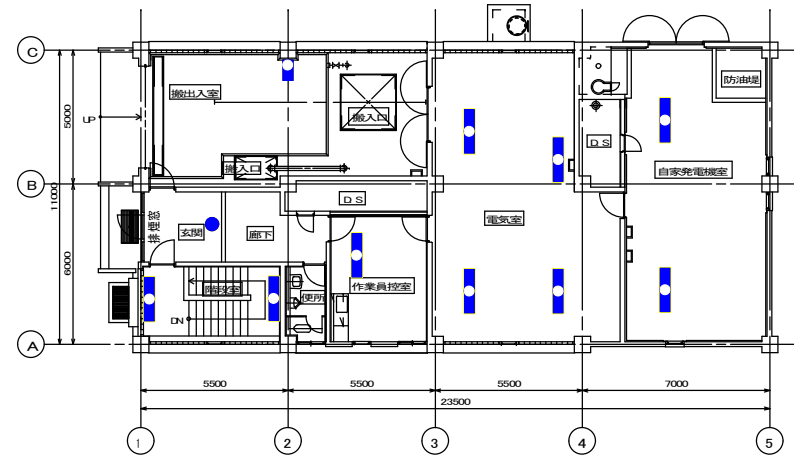
1階平面図 1/100
