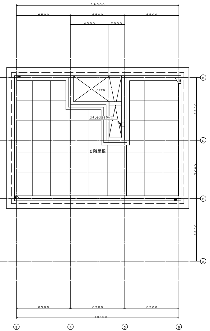
2階屋根平面図 S=1/100
