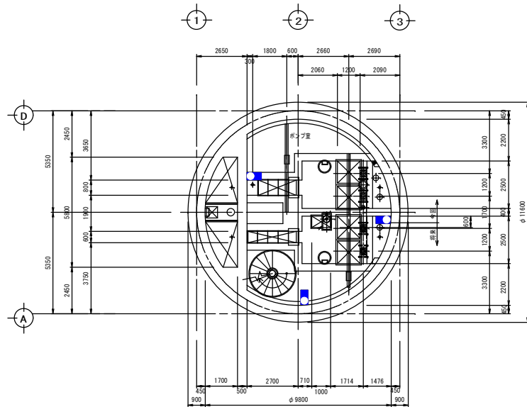
82F 平面図 S=1/100
