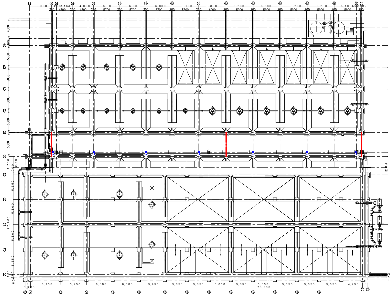
反応槽下層平面図 縮尺1/300
