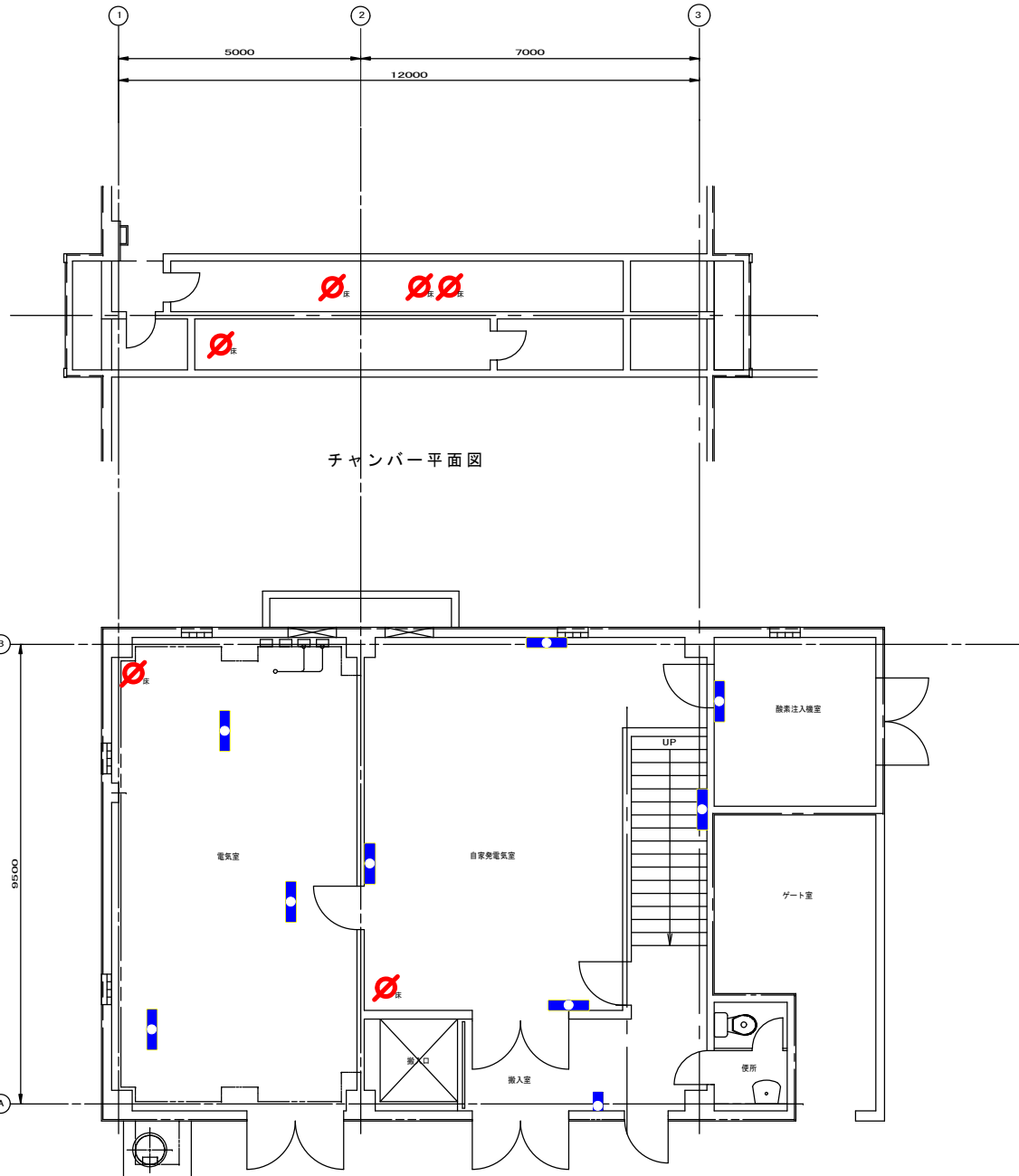
1階平面図
