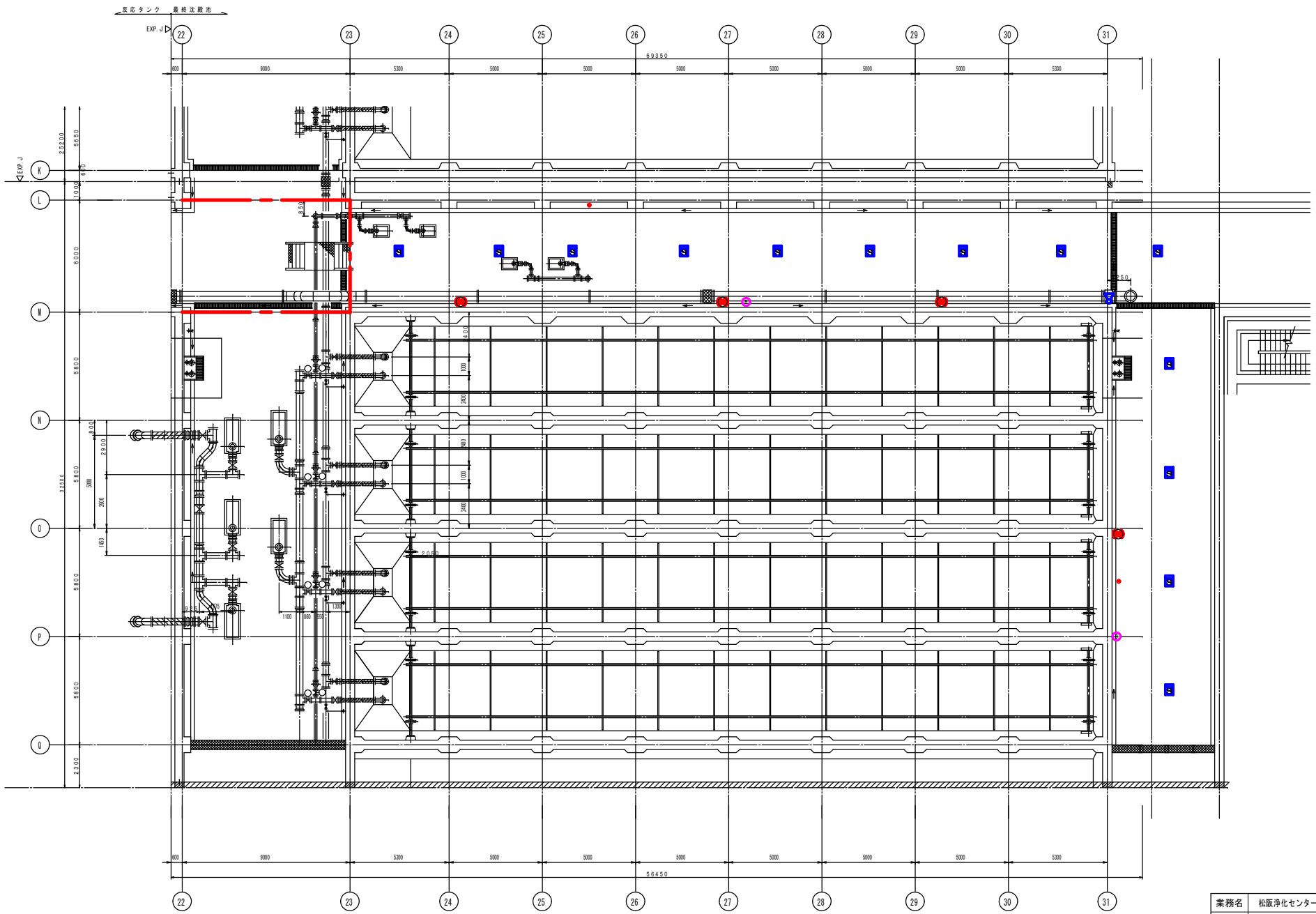
終沈下部平面図 S=1/200
