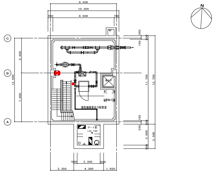
B 1階平面図 1/100
