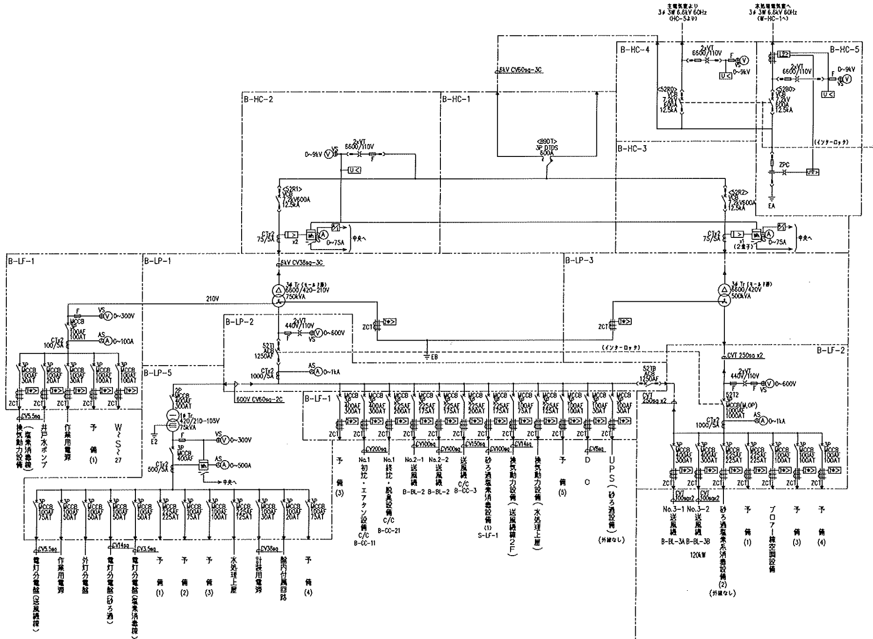
送風機単線結線図
