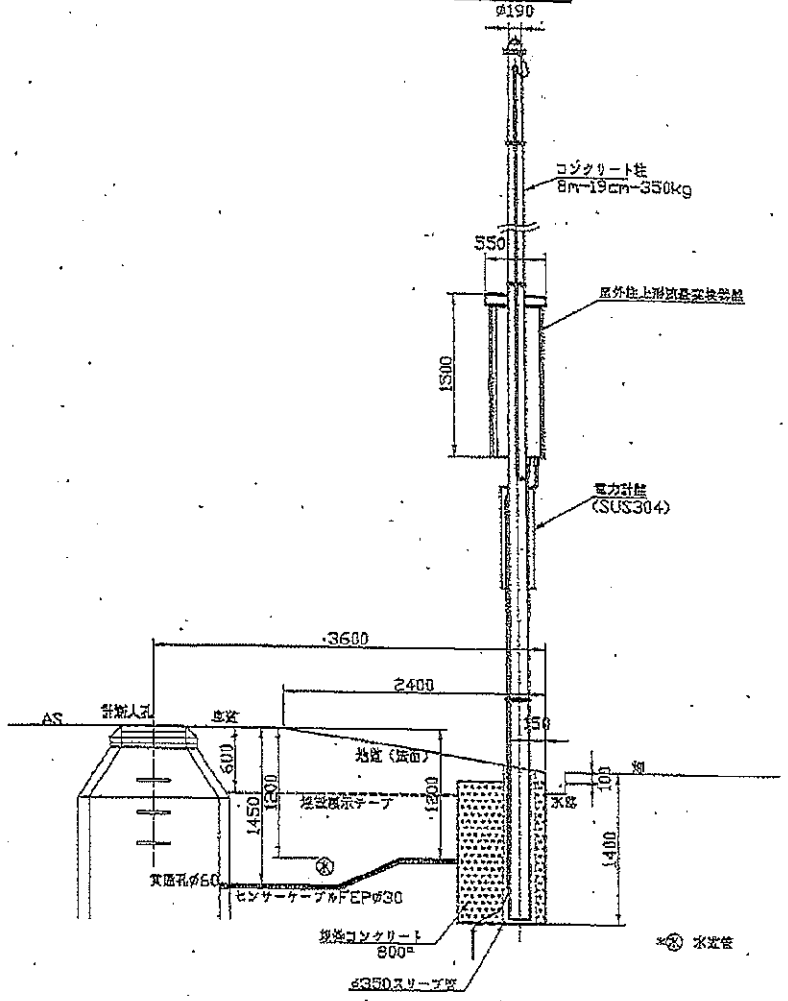
側面図
