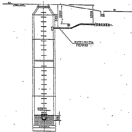
B-B 断面図
