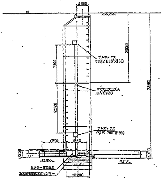
A-A 断面図
