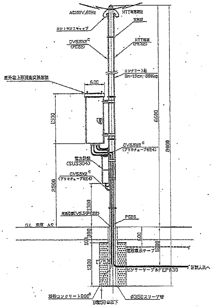
正面図
