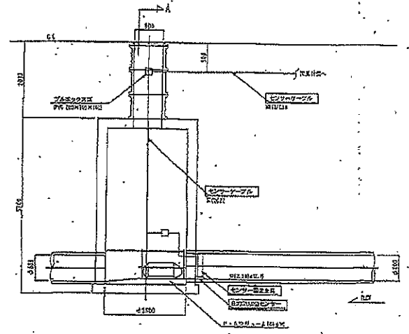
針測入孔部配線図 (S-1/10)
